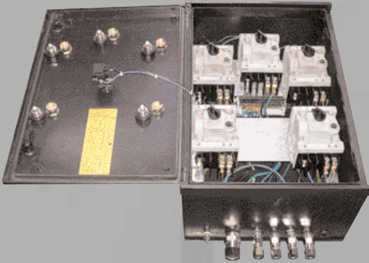
Armoire Marina de protection par disjoncteur.
