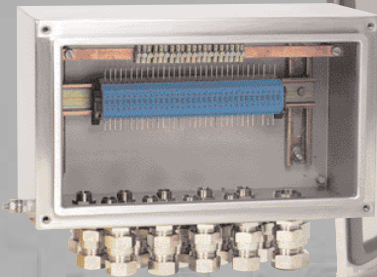
Bornier et boîte horizontale
