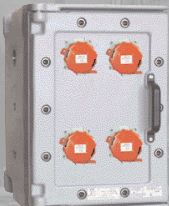
Coffret IIB aluminium équipé de 4 socles 3P+T 380/415V
